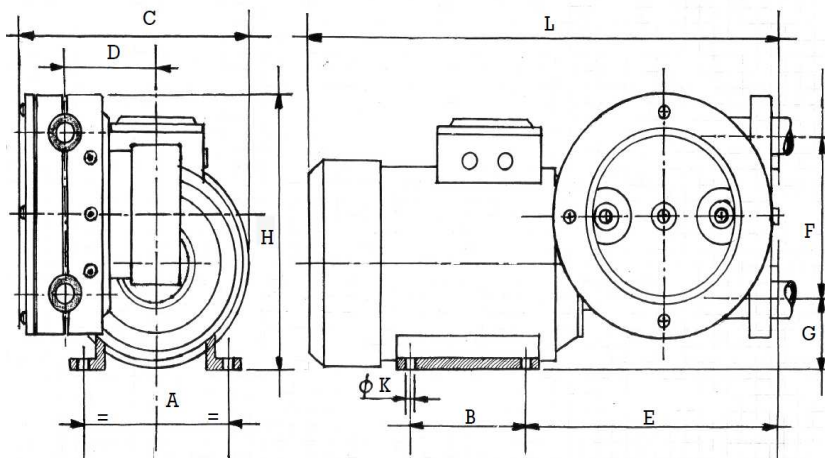
DIMENSIONI D'INGOMBRO POMPE PERISTALTICHE SERIE IPI 96 -150-300
